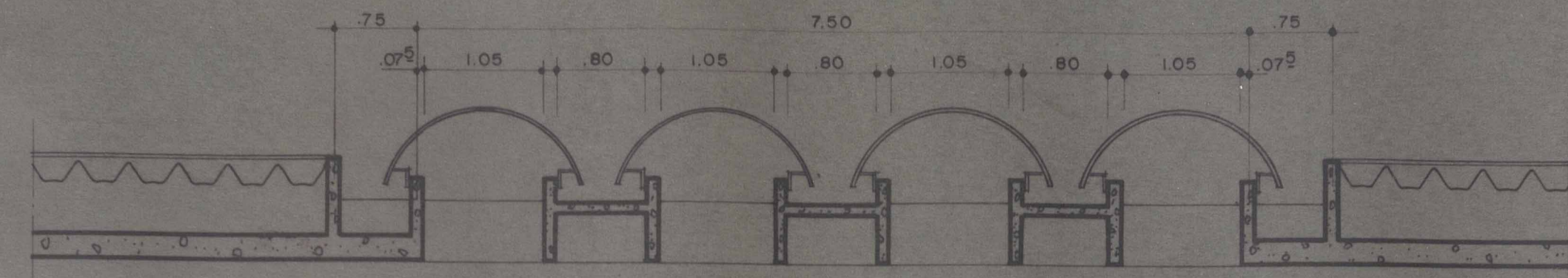
CORTE 1-1 ESC. 1:50
