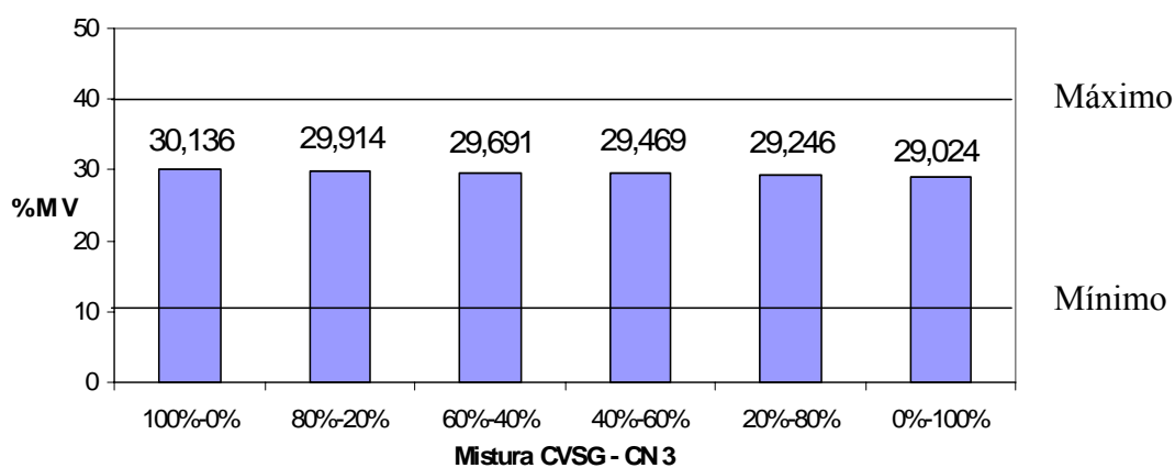
Figura 52. Valores médios percentuais dos teores de matérias voláteis das misturas de CVSG e CN3, com apresentação dos valores mínimos e máximos para operação no alto forno.
