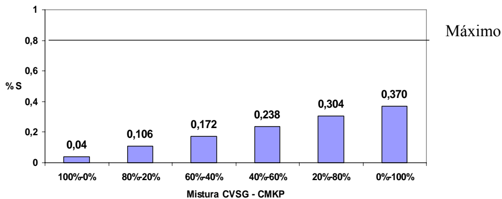
Figura 40. Valores médios percentuais dos teores de enxofre das misturas de CVSG e CMKP, com apresentação dos valores máximo para operação no alto forno.
