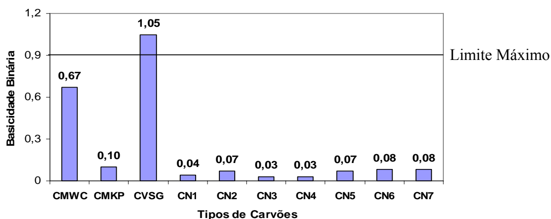
Figura 29. Valores das basicidades binárias das escórias no alto forno, estimada pela relação dos teores médios de \text{CaO} e de \text{SiO}_2 , considerando as respectivas massas moleculares e o limite máximo ideal para o alto forno.
