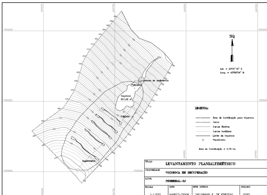
Figura 7: Levantamento planialtimétrico da voçoroca estudada em Pinheiral – RJ.
