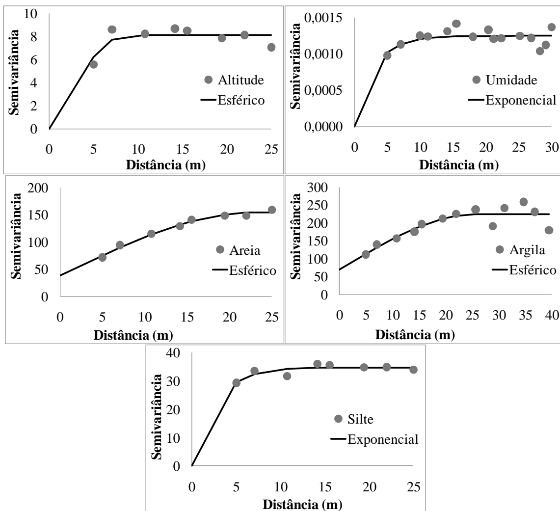
Figura 11: Semivariogramas experimentais da altitude e atributos físicos do solo.
