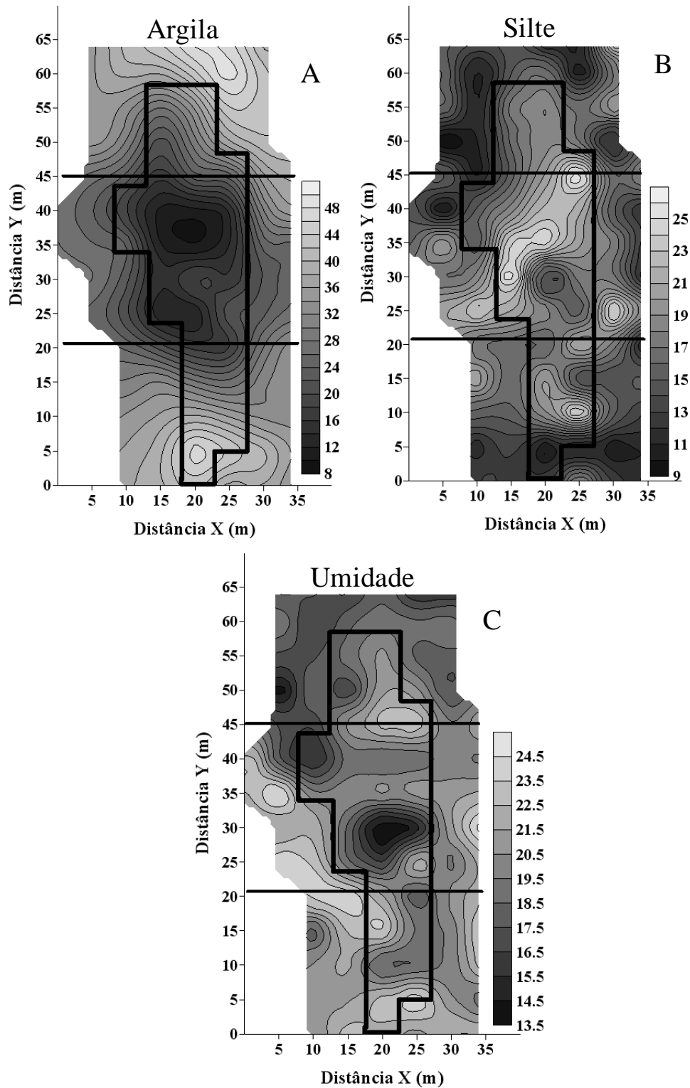
Figura 13: Mapas de variabilidade espacial: A) Argila ( \text{g kg}^{-1} ); B) Silte ( \text{g kg}^{-1} ); C) Umidade gravimétrica ( \text{g kg}^{-1} ).
