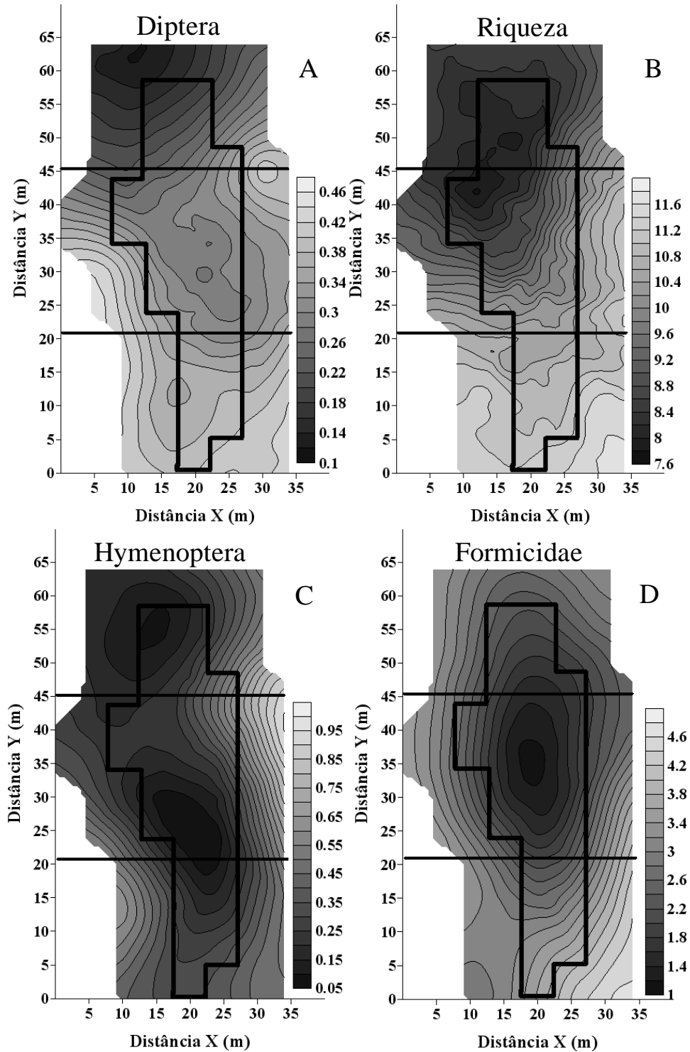
Figura 22: Mapas de variabilidade espacial: A) Diptera ( \text{ind arm}^{-1} \text{dia}^{-1} ); B) Riqueza; C) Hymenoptera ( \text{ind arm}^{-1} \text{dia}^{-1} ); D) Formicidae ( \text{ind arm}^{-1} \text{dia}^{-1} ).
