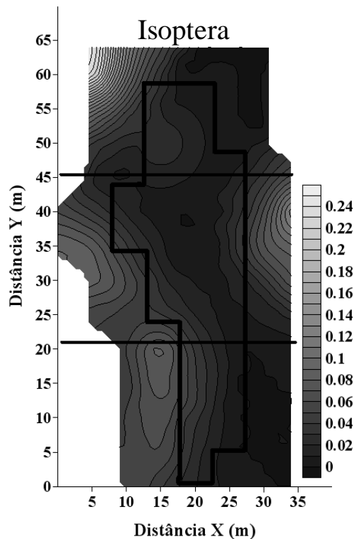
Figura 24: Mapa de variabilidade espacial de Isoptera ( \text{ind arm}^{-1} \text{ dia}^{-1} ).
