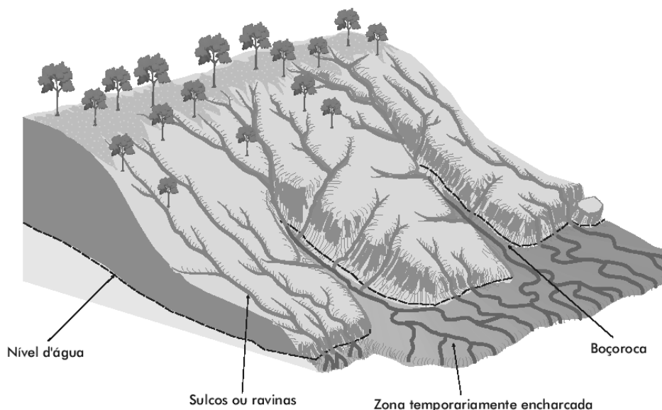
Figura 2: Morfologia de sulcos e voçorocas. Retirado de KARMANN (2003).
