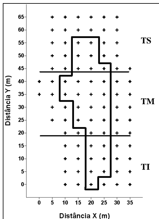
Figura 9: Grade regular dos pontos amostrados. TS: terço superior da voçoroca; TM: terço médio da voçoroca; TI: terço inferior da voçoroca. A área delimitada diferencia o entorno do interior da voçoroca.
