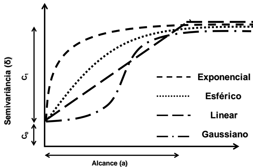
Figura 5: Modelos de ajuste de semivariogramas. C_0 : efeito pepita; C_1 : variância estrutural; a : alcance.
