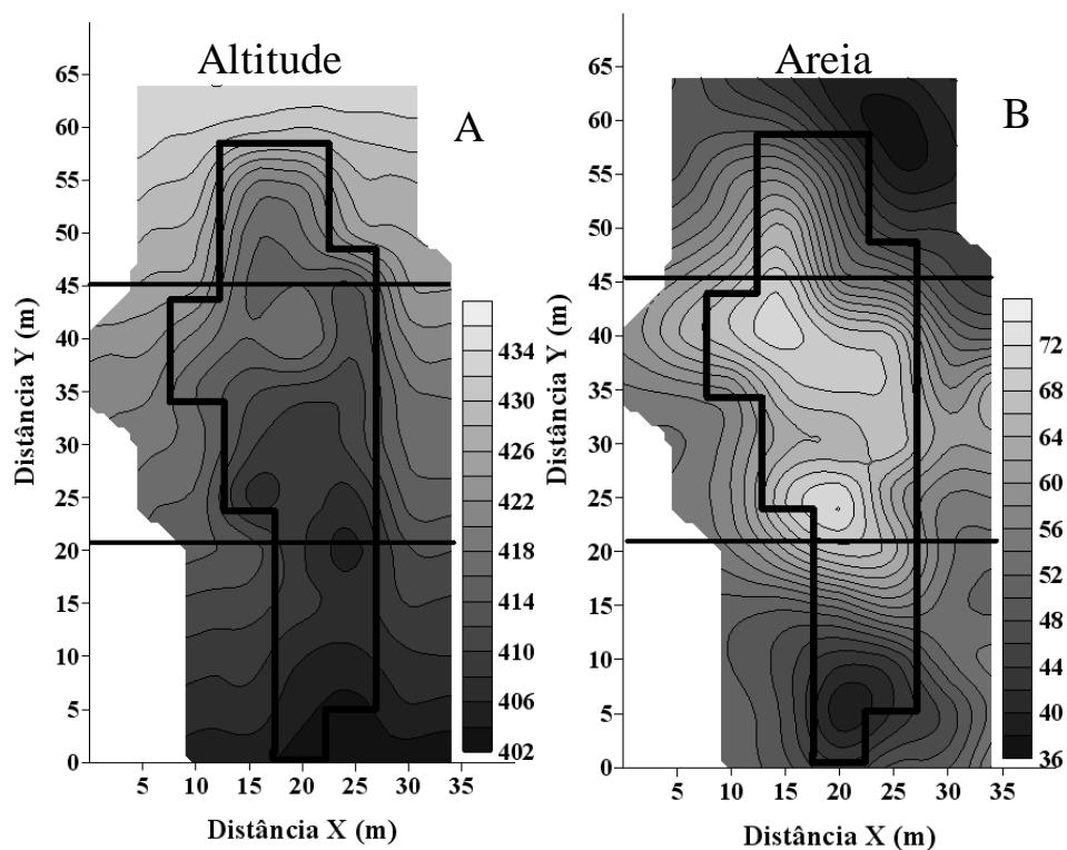
Figura 12: Mapas de variabilidade espacial: A) Altitude (m); (B) Areia ( \text{g kg}^{-1} ).
