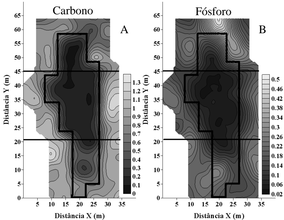
Figura 18: Mapas de variabilidade espacial: A) Carbono orgânico (%); B) Fósforo ( \text{mg dm}^{-3} ).
