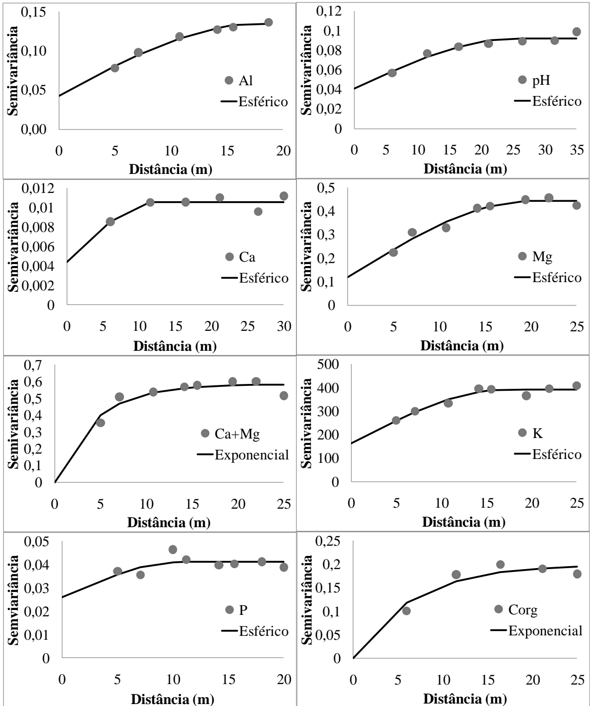
Figura 14: Semivariogramas dos atributos químicos do solo. Al: alumínio ( \text{cmol}_c \text{dm}^{-3} ); pH: potencial hidrogeniônico (1:2,5); Ca: cálcio ( \text{cmol}_c \text{dm}^{-3} ); Mg: magnésio ( \text{cmol}_c \text{dm}^{-3} ); K: potássio ( \text{mg kg}^{-1} ); P_{\log} : logaritmo do fósforo ( \text{mg dm}^{-3} ); C_{\text{org}} : carbono orgânico ( \text{g kg}^{-1} ).
