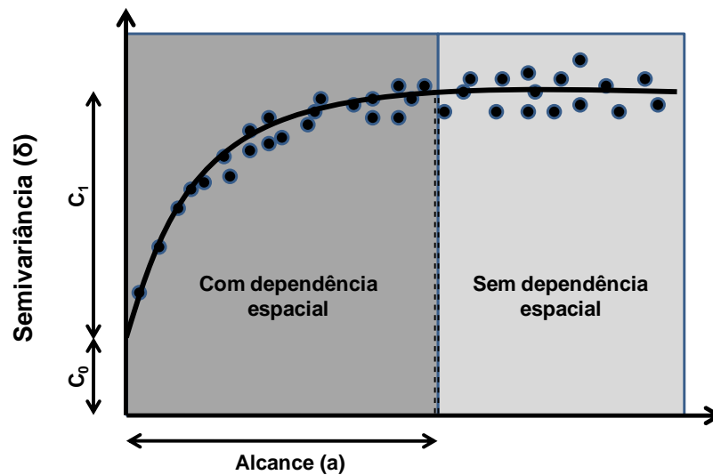
Figura 4: Parâmetros do semivariograma: C_0 : efeito pepita; C_1 : variância estrutural; C_0 + C_1 : patamar; a : alcance.
