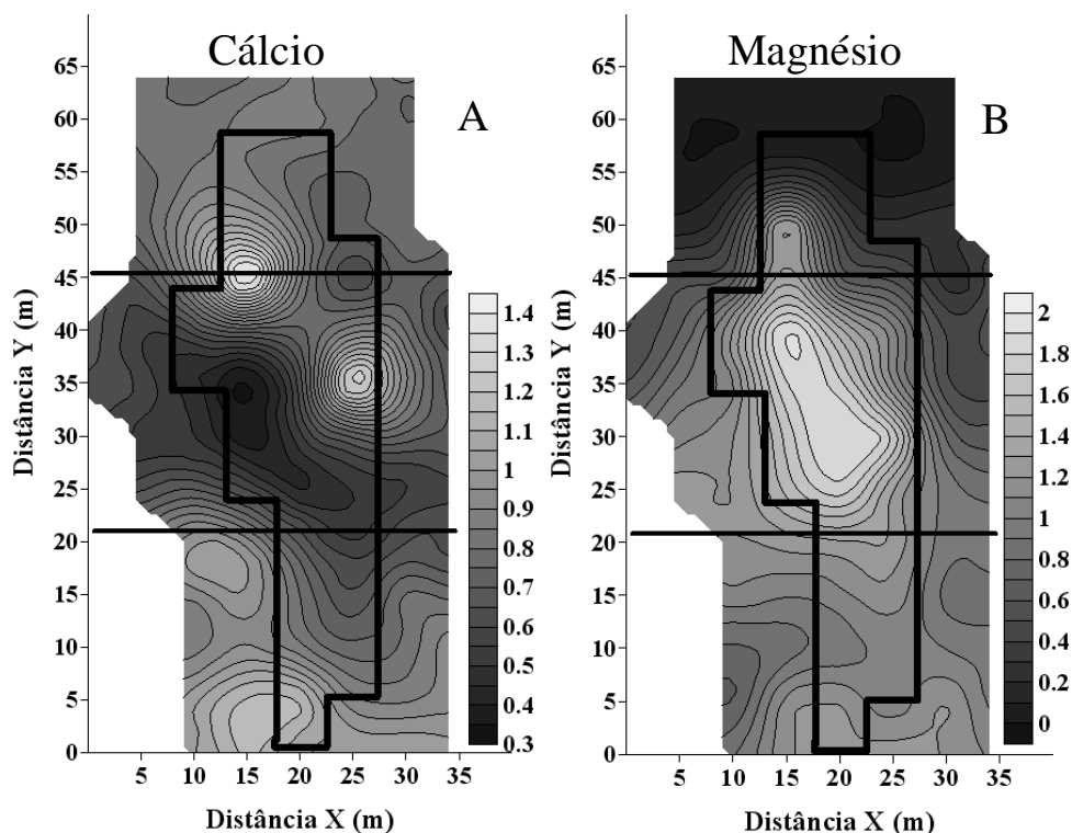
Figura 16: Mapas de variabilidade espacial A) Cálcio ( \text{cmol}_c \text{ dm}^{-3} ); B) Magnésio ( \text{cmol}_c \text{ dm}^{-3} ).
