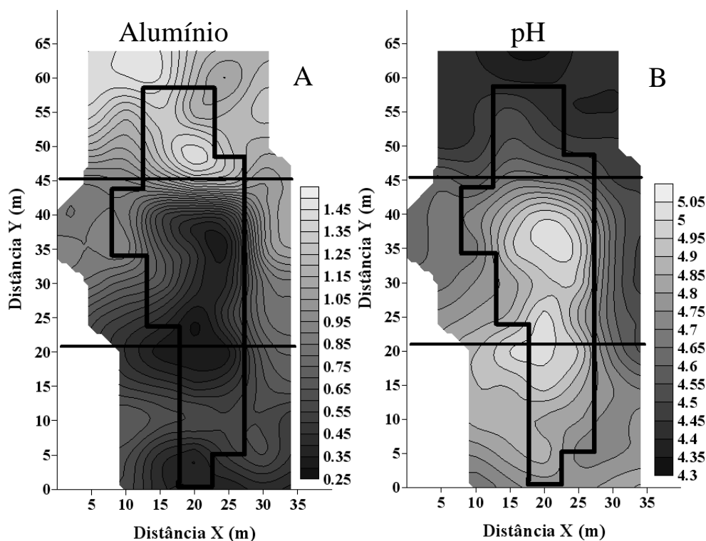
Figura 15: Mapas de variabilidade espacial: A) Alumínio ( cmol_c dm^{-3} ); B) pH (1:2,5).
