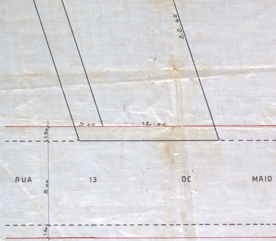
PLANTA 1: 200
